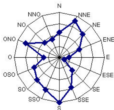
Distribution de la direction du vent (période de navigation avril à octobre)
